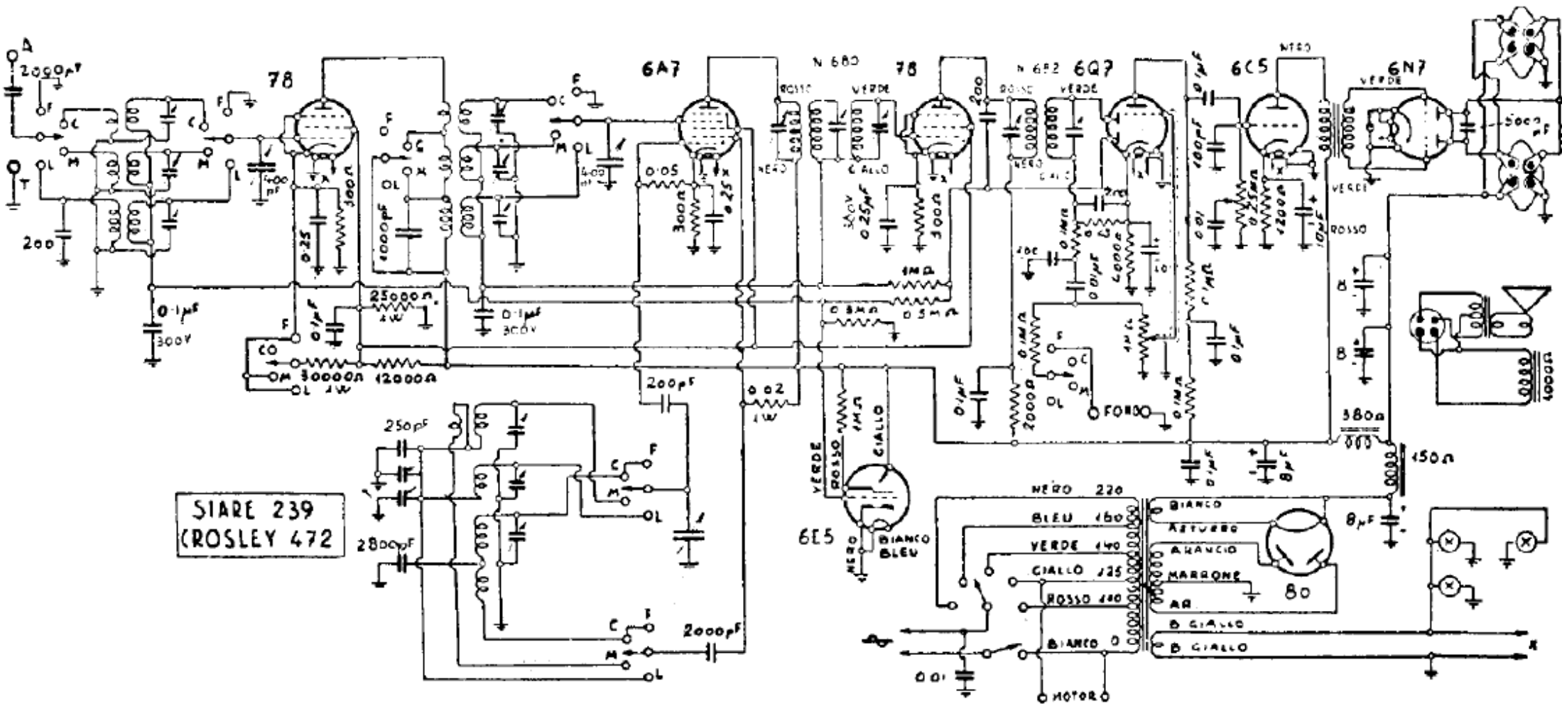
RADIO SIARE. — Modelli « Siare 239 » e « Crosly 472 » a onde corte medie e lunghe; con sintetizzatore visivo a tubo a raggi catodici (6E5). - Produzione 1937. - Media frequenza: 468 kHz.
